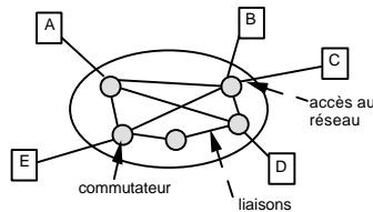
Réseau à commutation
