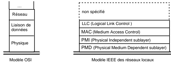
Modèle en couches des réseaux locaux
