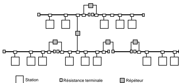
Exemple de réseau IEEE 802.3
