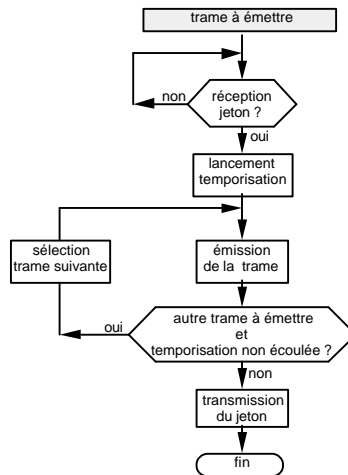
Principe général de l'accès par jeton
