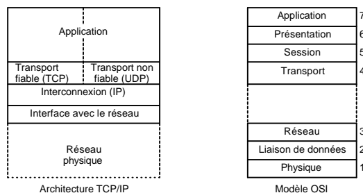
Architectures en couches TCP/IP et OSI
