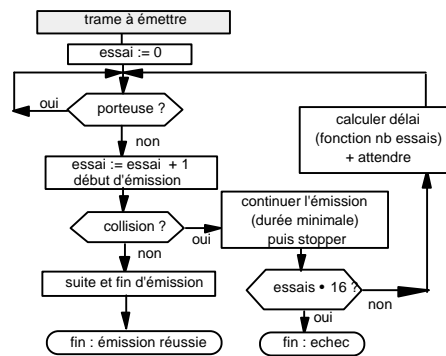
Algorithme d'émission CSMA/CD
