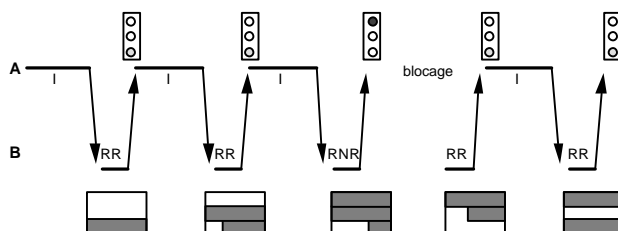
Mécanisme du contrôle de flux
