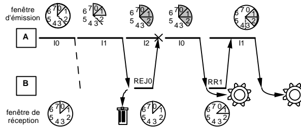
Scénario d'un protocole Go-back-N
